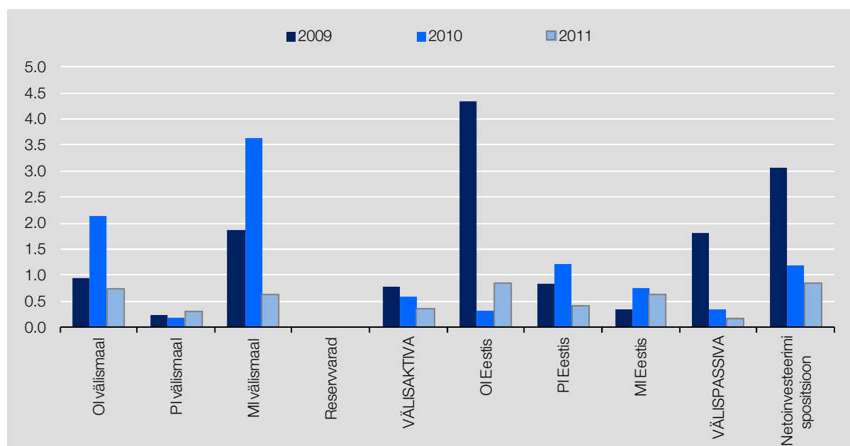
Joonis 37. Investeerimispositsiooni korrigeerimine (MAPE, % esialgsest väärtusest)
