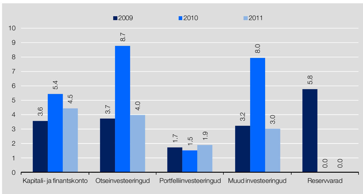
Joonis 20. Finantskonto korrigeerimine (RMSRE, % aegrea volatiilsusest)
