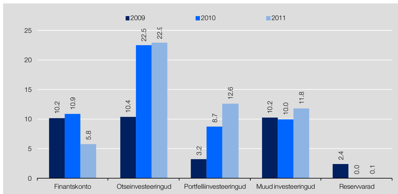
Joonis 2. Maksebilansi kiirhinnangu finantskonto korrigeerimine (RMSRE, % aegrea volatiilsusest)
